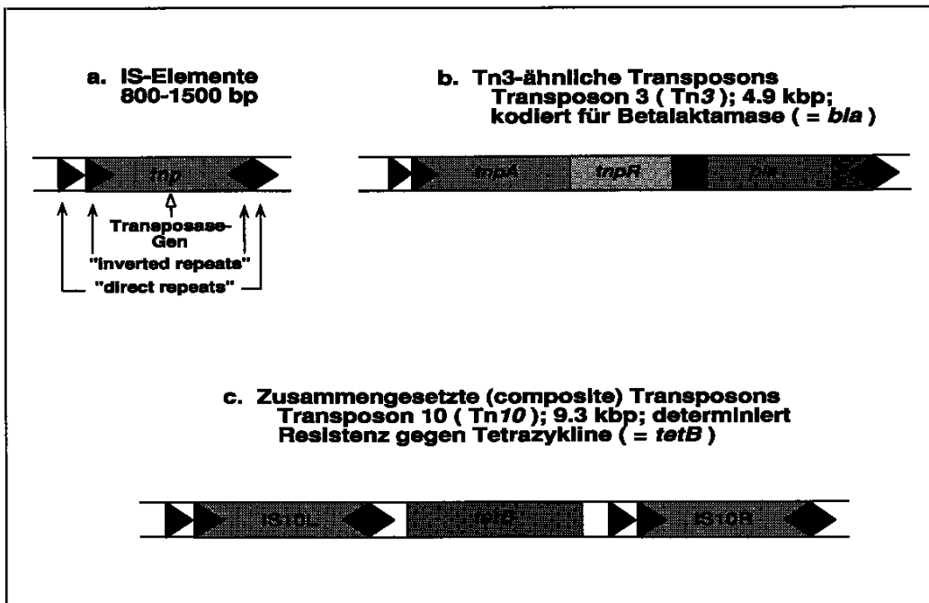
Abbildung 2: Transponierbare DNS-Elemente
