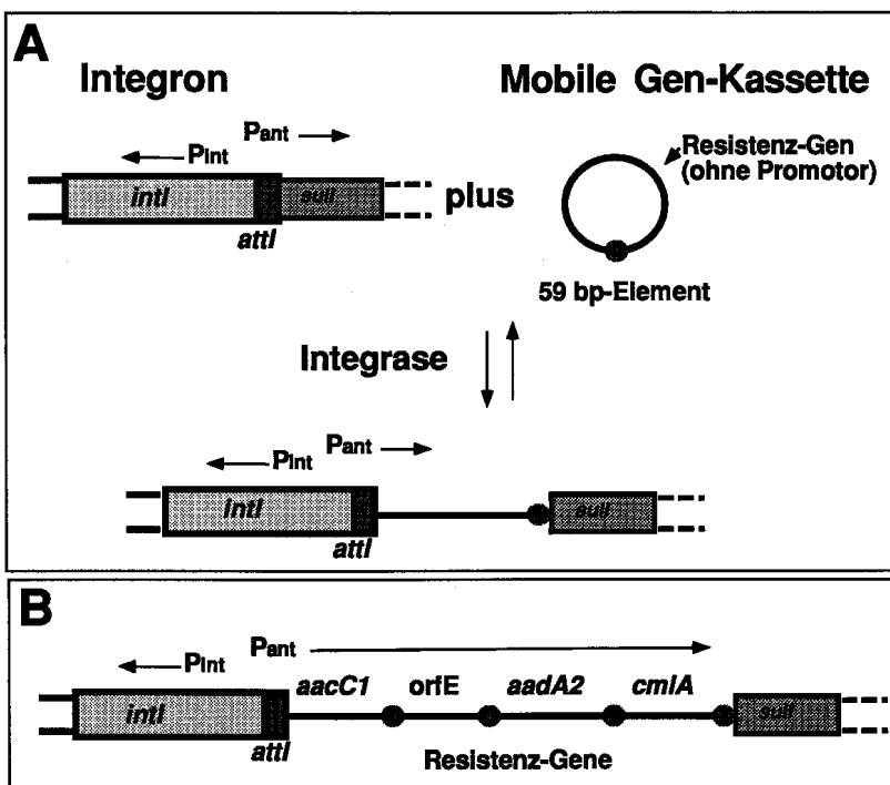
Abbildung 1: Das Integron-Konzept
